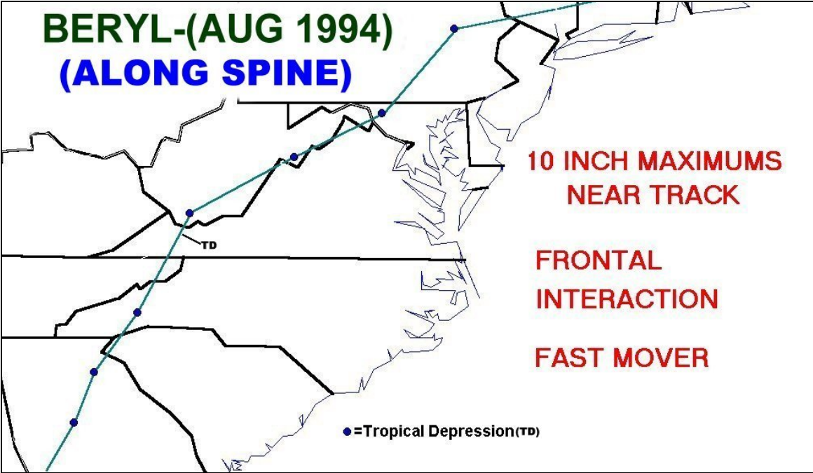
Fig. A-106: August 16-18, 1994. BERYL .
